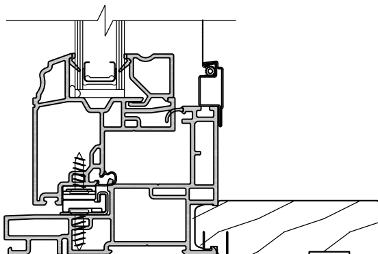
JAMB EXTENSIONS
