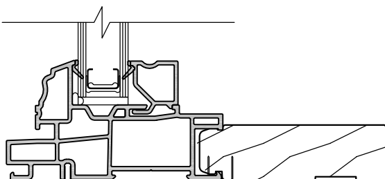
JAMB EXTENSIONS
