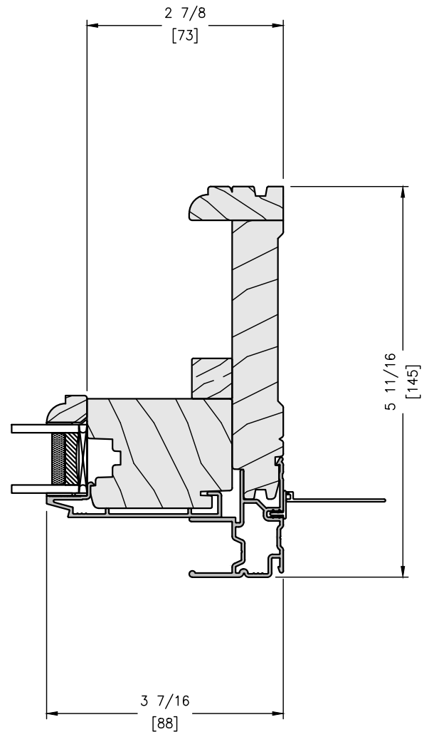
FIXED JAMB
