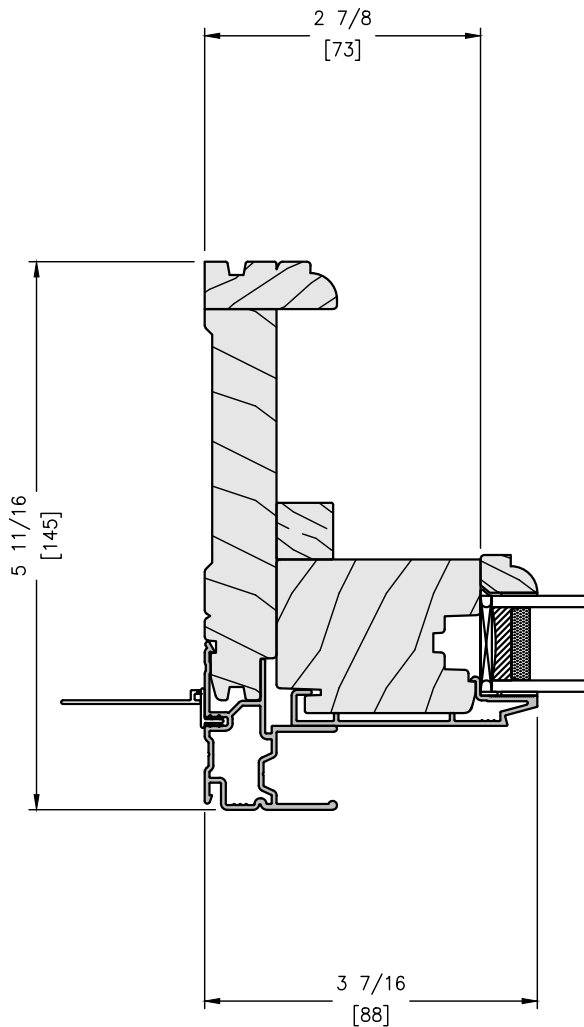
FIXED JAMB
