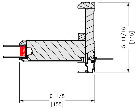
FIXED JAMB
