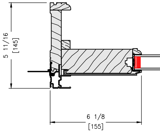
FIXED JAMB
