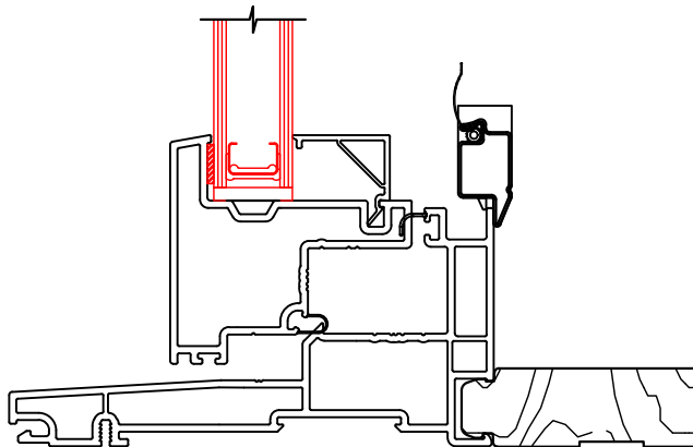
JAMB EXTENSIONS
