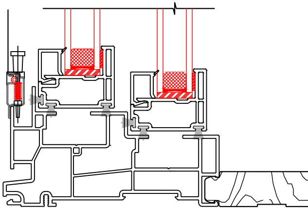
JAMB EXTENSIONS
