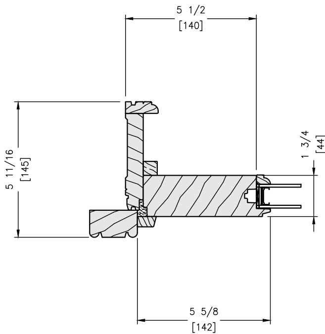
FIXED JAMB
